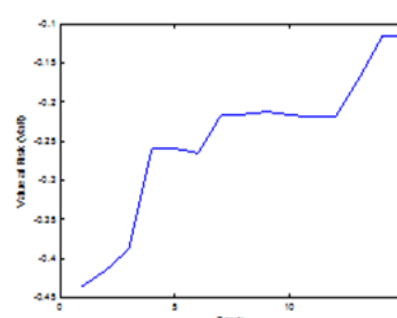
Figure-1.6. VaR.
